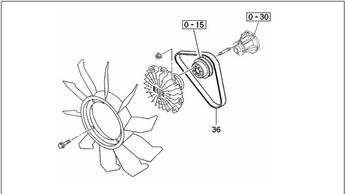
FIG.NO : 0-33 FAN AND FAN BELT
