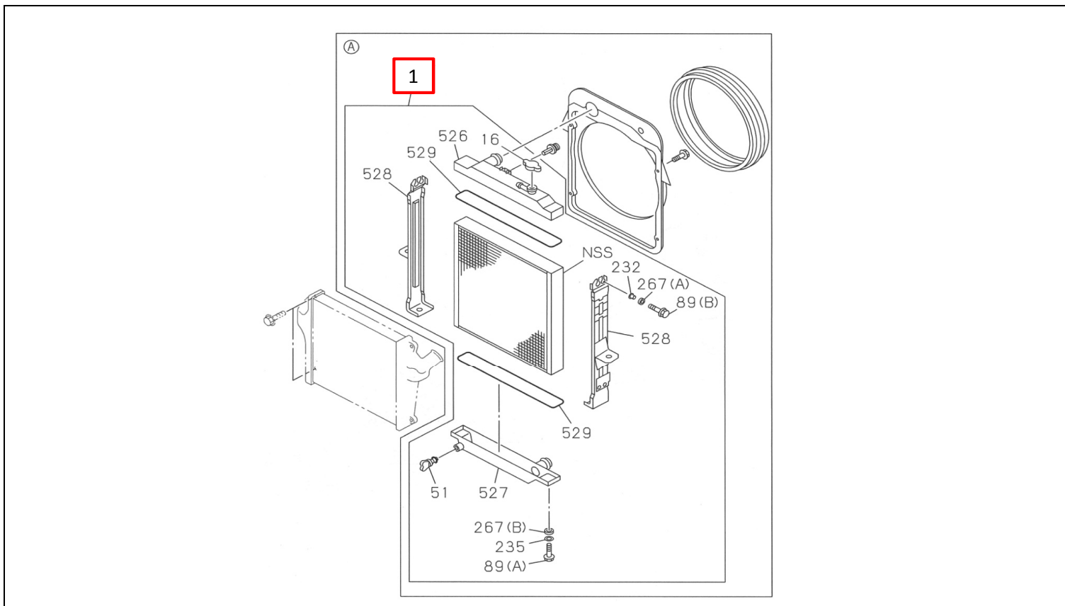
FIG.NO : 1-10 RADIATOR
