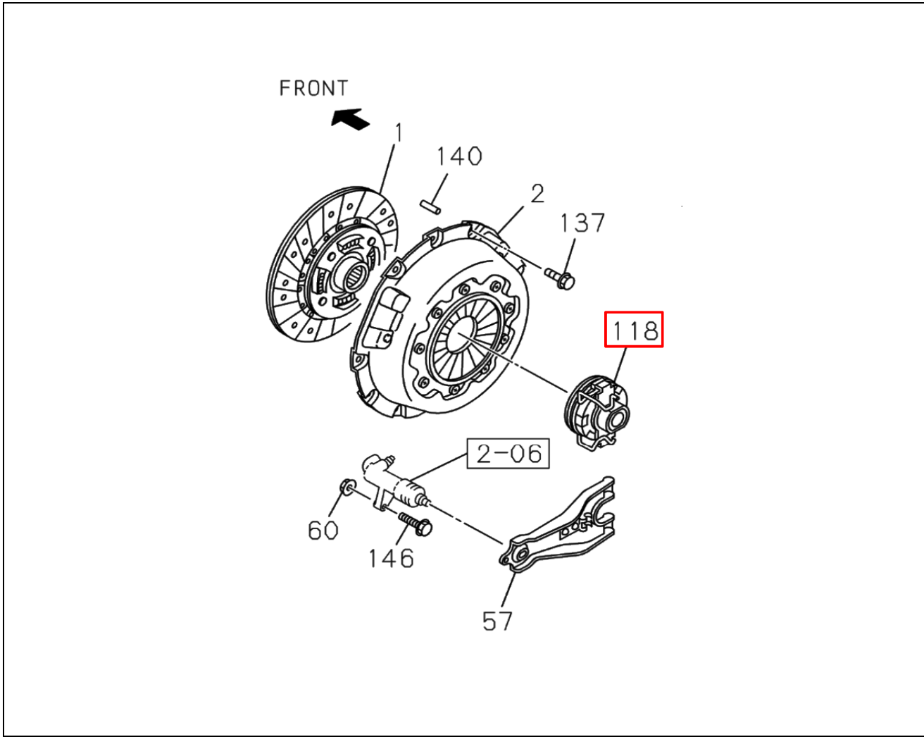
FIG NO : 2-01 CLUTCH
