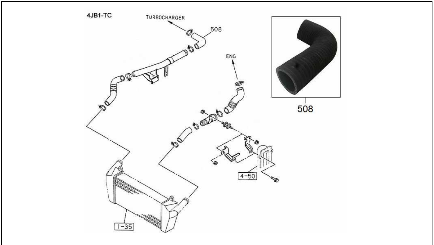
FIG.NO : 1-31 AIR DUCT
