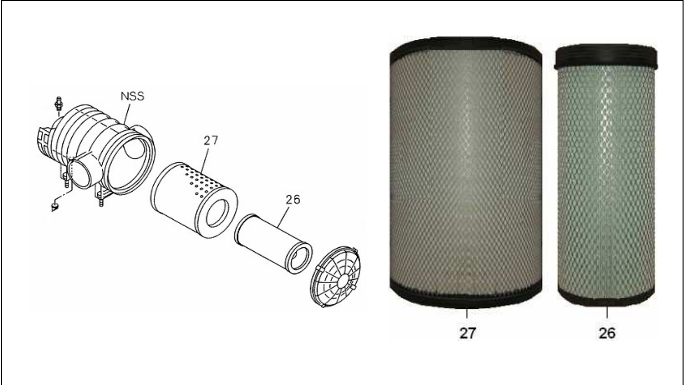
FIG.NO : 1-30 AIR CLEANER
