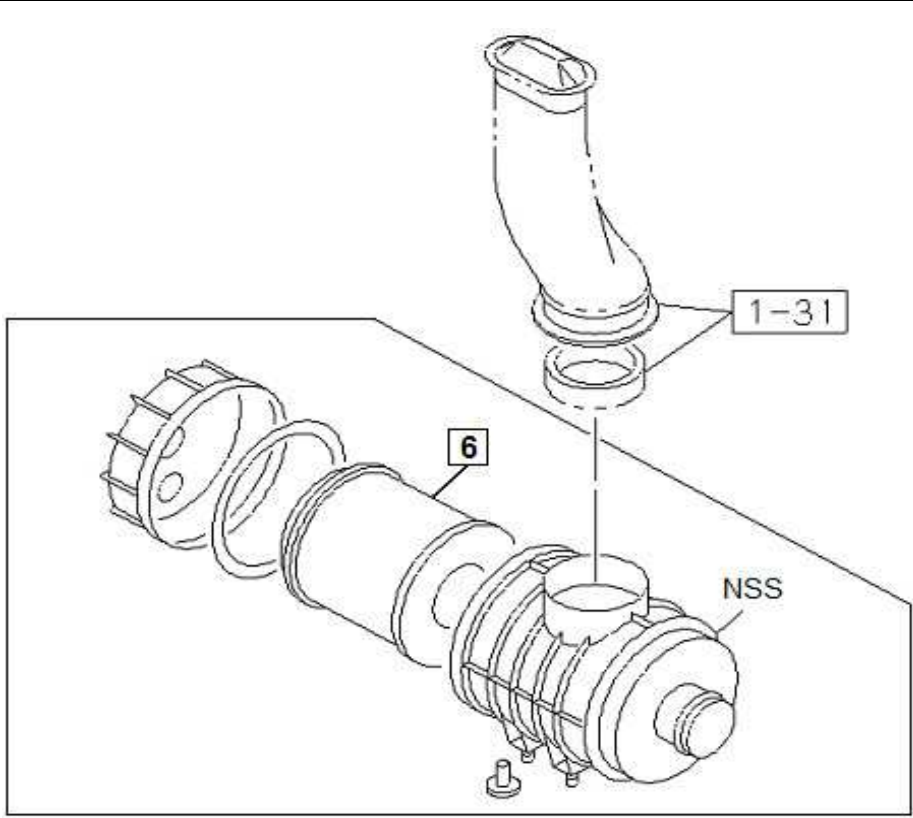
FIG.NO : 1-30 AIR CLEANER
