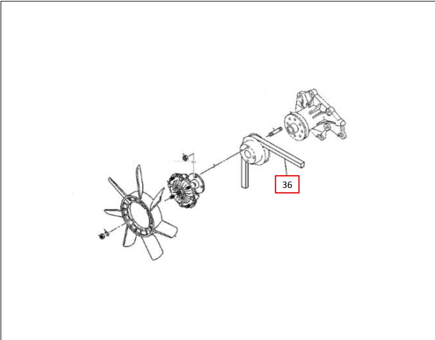
FIG NO : 0-33 FAN AND FAN BELT
