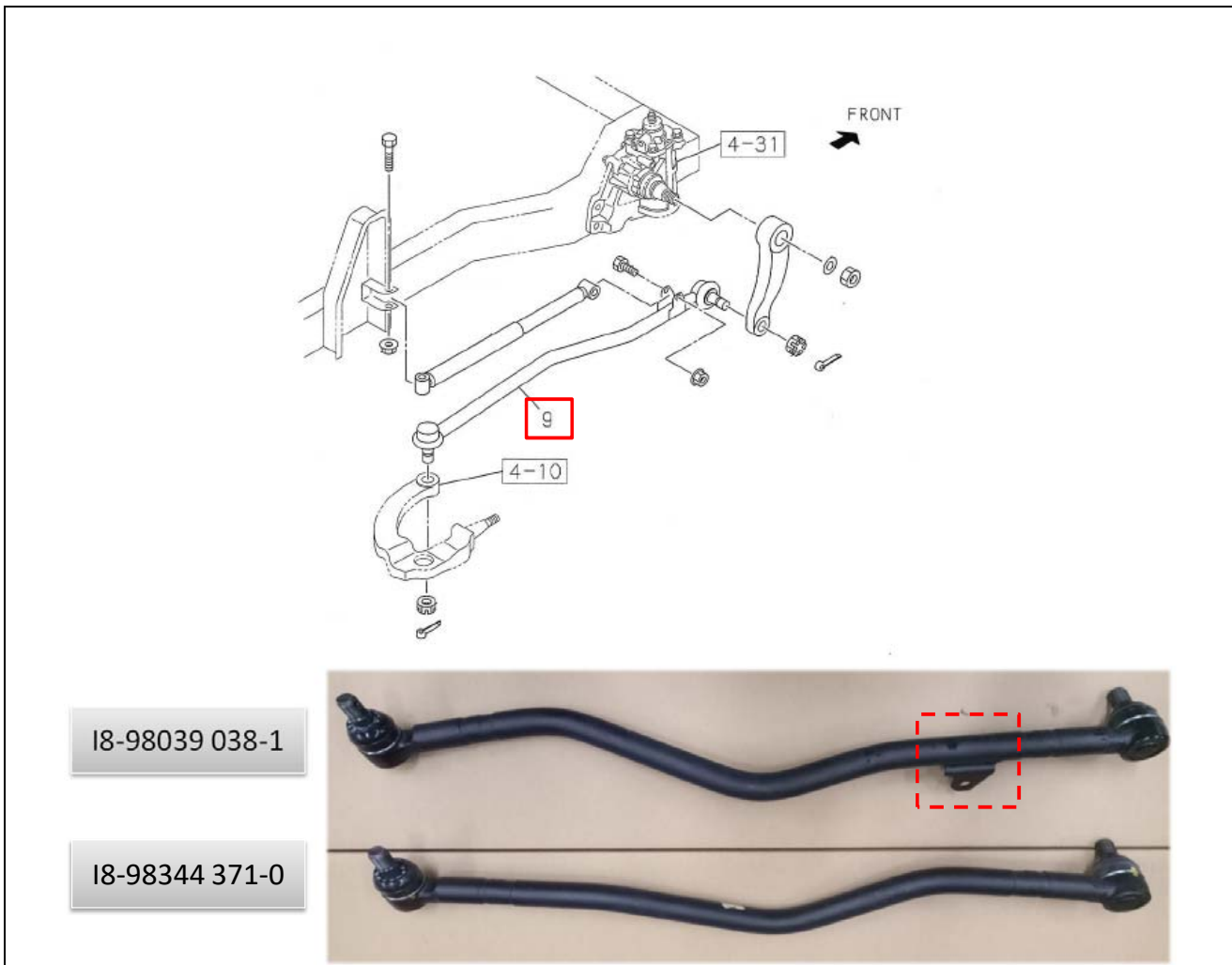
FIG NO : 4-33 STEERING LINKAGE
