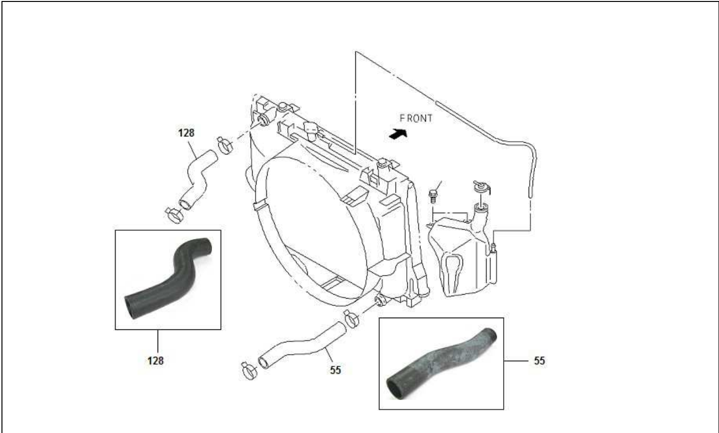
FIG.NO : 1-11 RADIATOR HOSE
