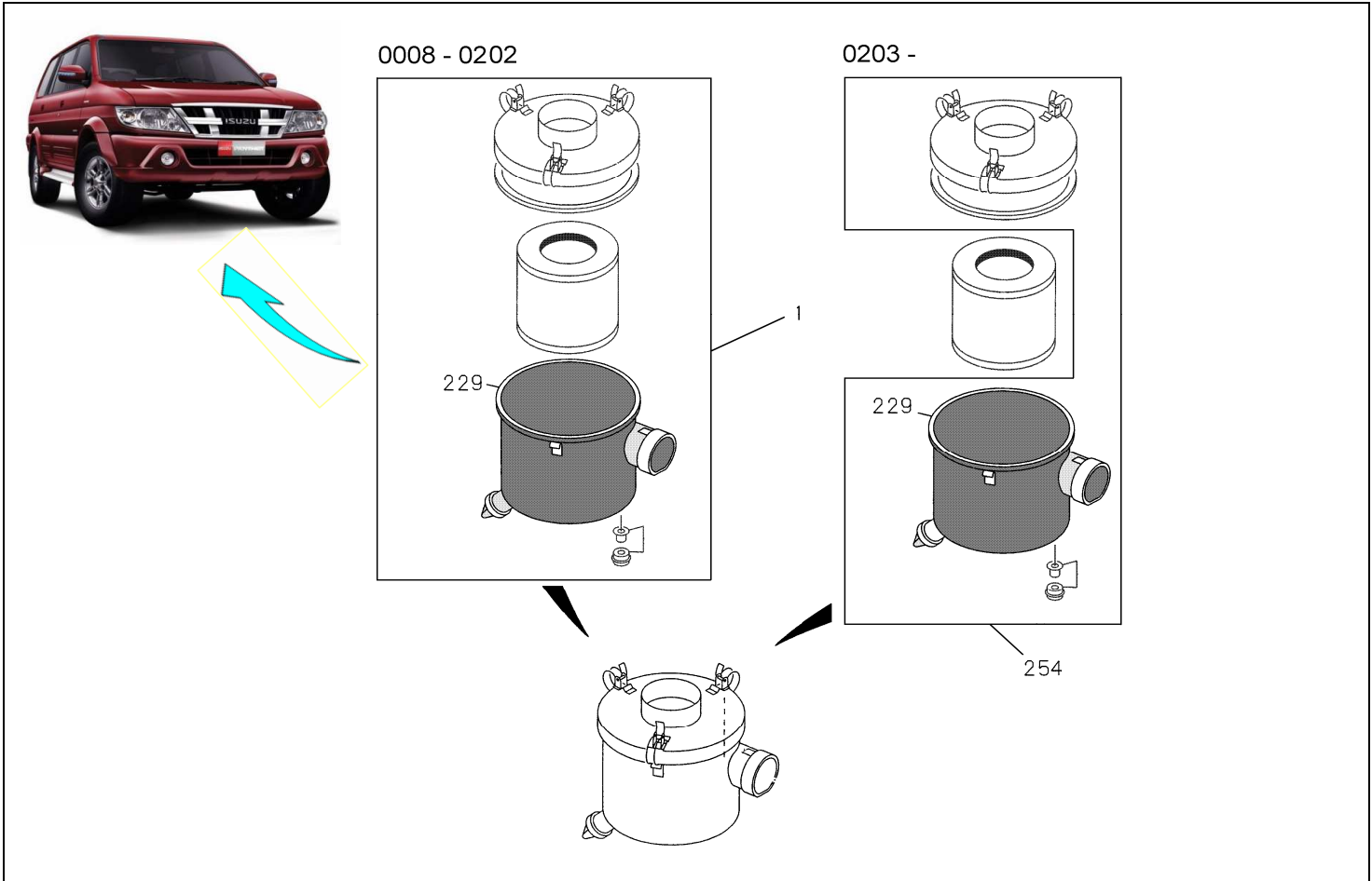
FIG.NO : 1-30 AIR CLEANER
