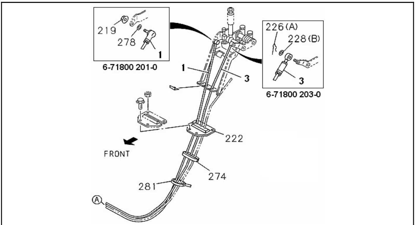
FIG.NO : 2-36 CABLE SHIFT & SELECT
