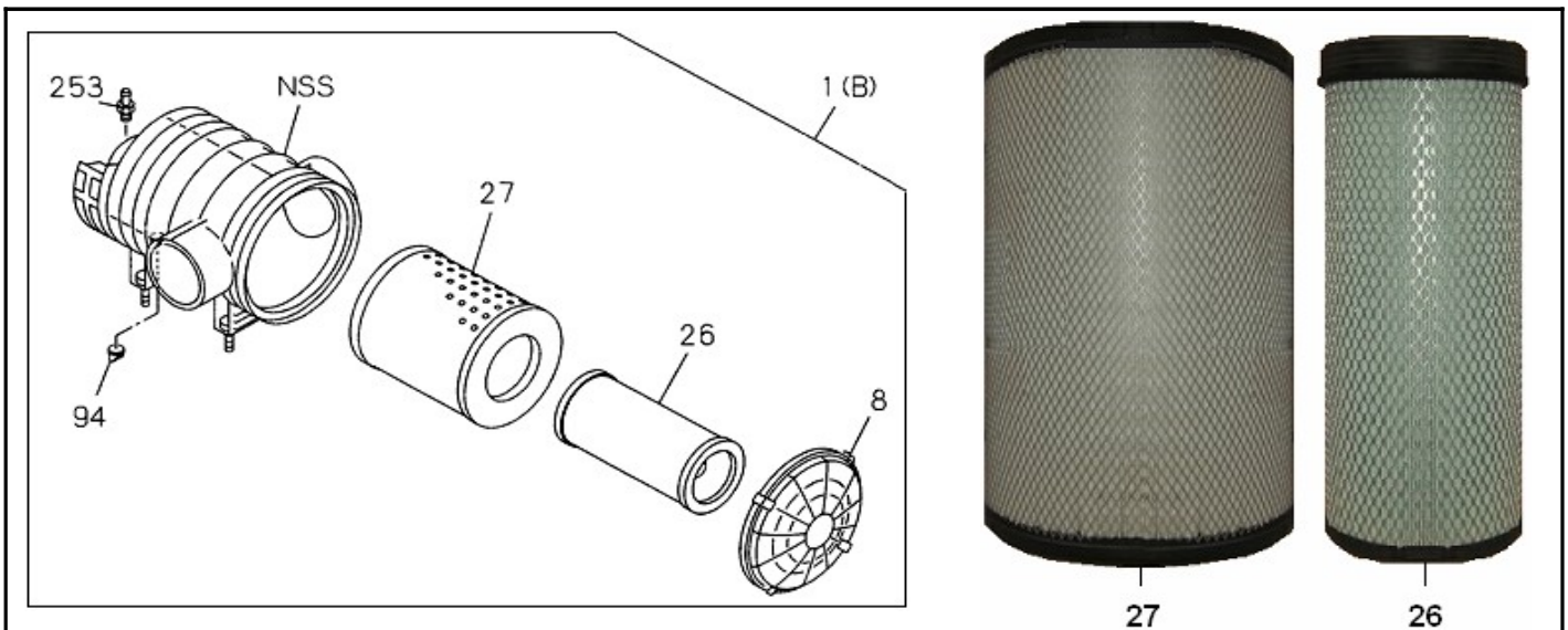
FIG.NO : 1-30 AIR CLEANER
